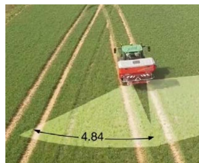
Система безступінчатого регулювання робочої ширини і «посекційного» відключення
